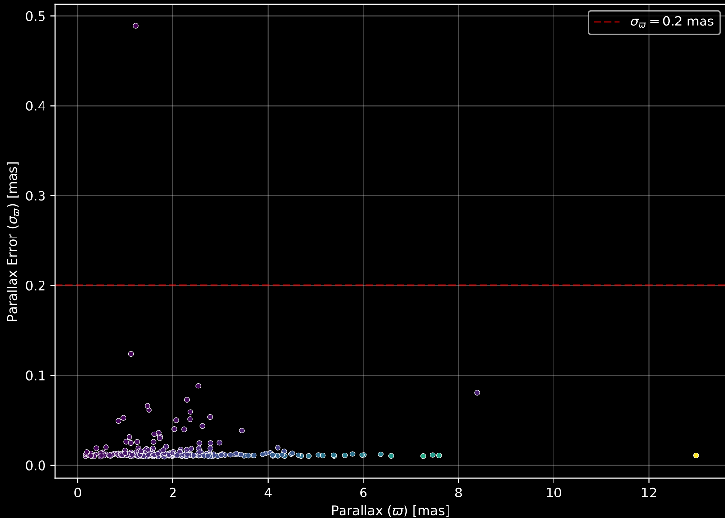
GALAH DR4 Field: [76] Parallax Quality (n= 301)
